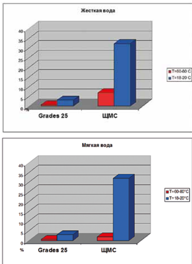
Рис. 1. Сравнение относительной площади загрязнения поверхности после промывки щелочным составом «Grades 25» и ЩМС (щелочным моющим средством)
